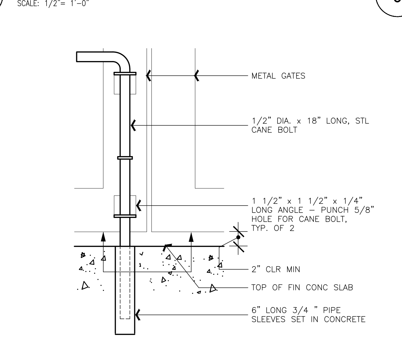
CANE BOLT SECTION SCALE: 3" = 1'-0"
