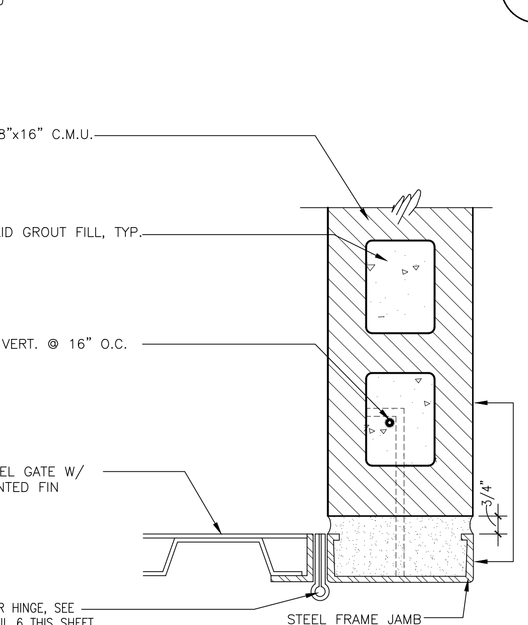
GATE JAMB SCALE: 3" = 1'-0"
