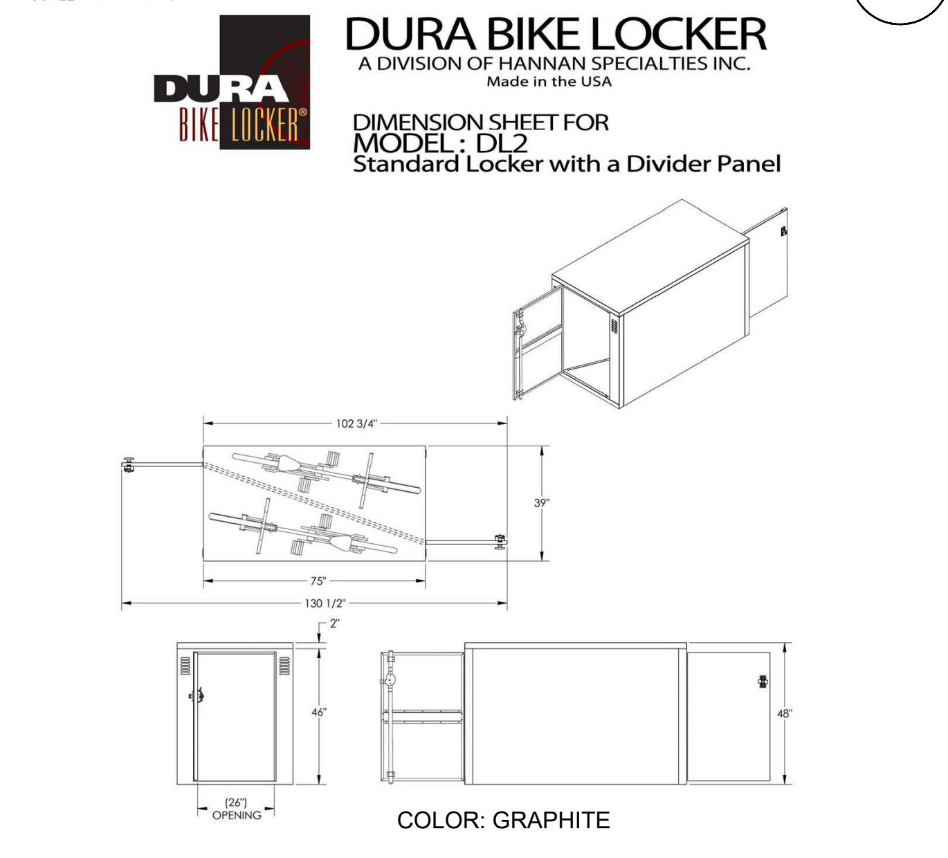
BIKE LOCKER - DOUBLE SCALE: N.T.S.
