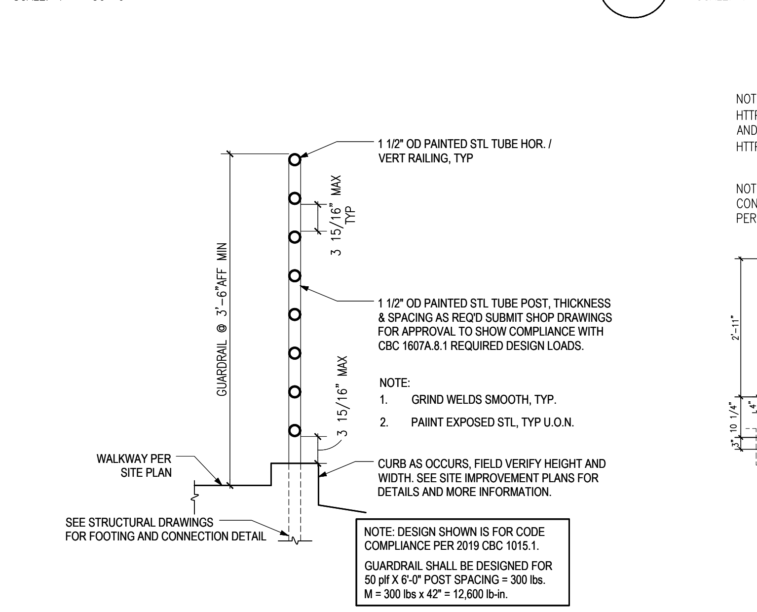
GUARDRAIL SCALE: 1" = 1'-0"
